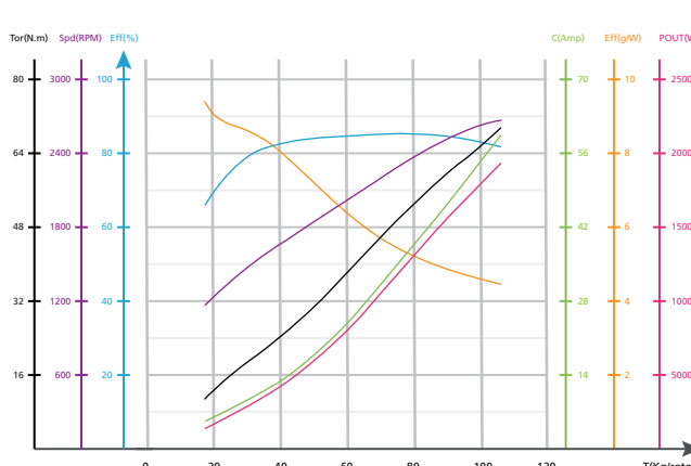
54*23"-11KV Load performance parameters
