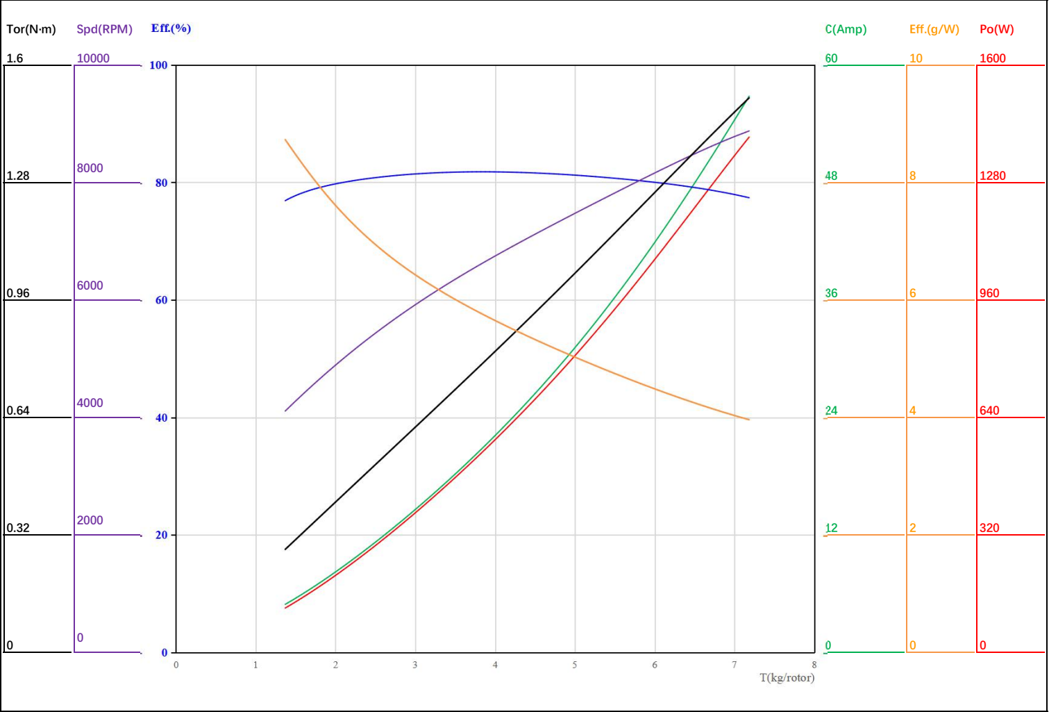
拉力数据表 Motor Propeller Pull Test Data
