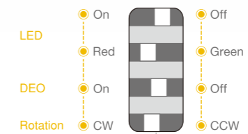
拨码开关设计
