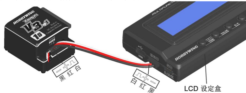
图 1 XERUN V3 电调和 LCD 设定盒的连接
