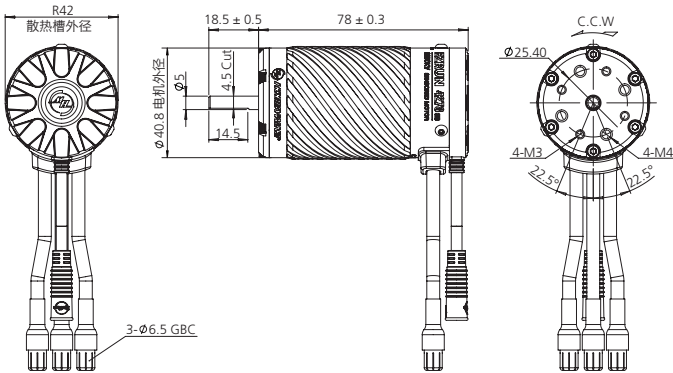
EZRUN 4278SD G2R
