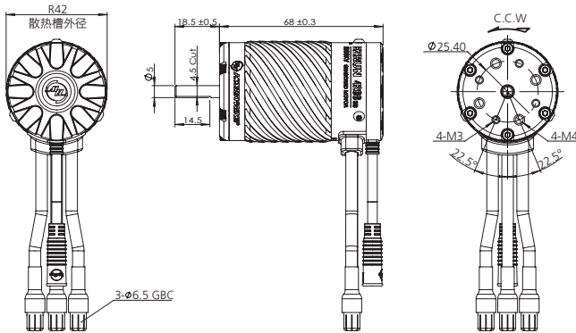
EZRUN 4268SD G2R
