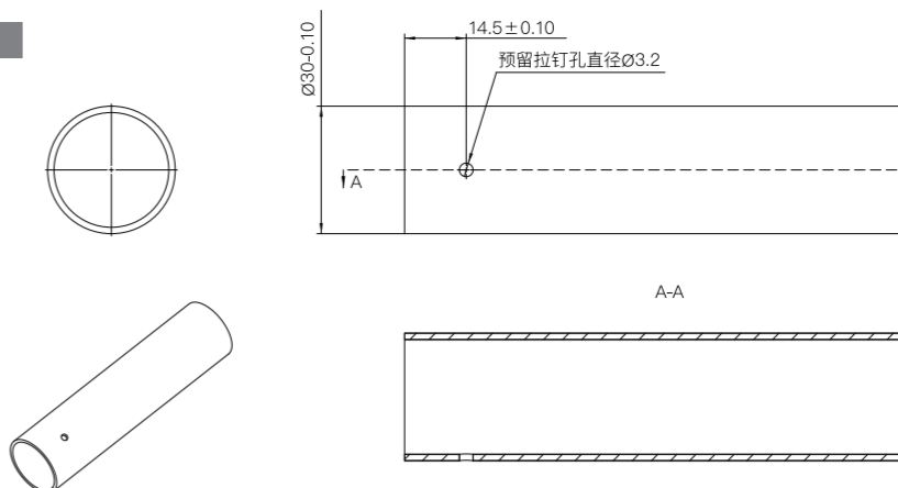
D30-碳管加工示意图
