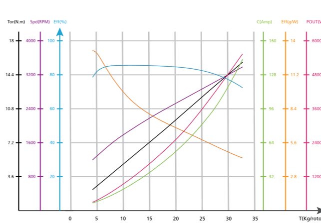
X11 G2-54V拉力负载曲线图
