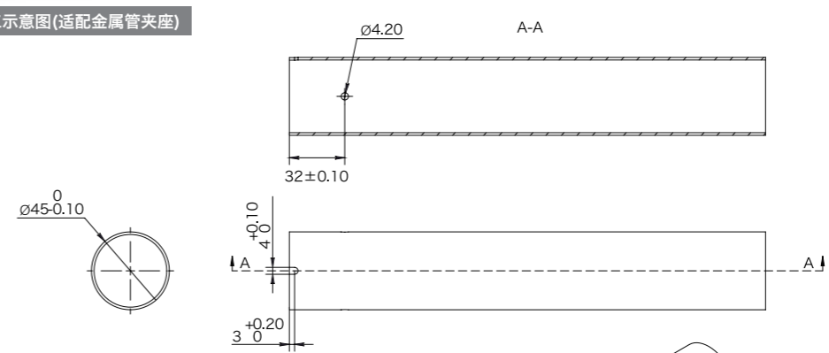
D45-碳管加工示意图 (适配金属管夹座)
