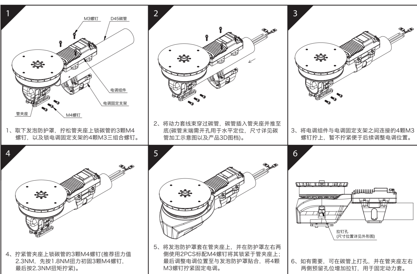
D45用户安装示意图 (适配金属管夹座)
