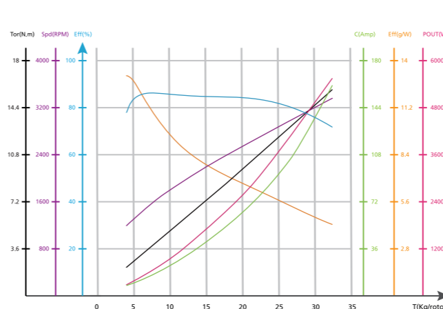
X11 G2-48V拉力负载曲线图
