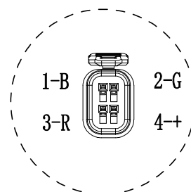
接线示意图
